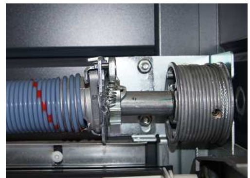
Porte de garage à torsion - Système de pose rapide Crédit photo : VENDÔME
